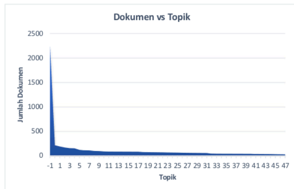
38 Gambar 4.10 Grafik Distribusi Topik pada dokumen
