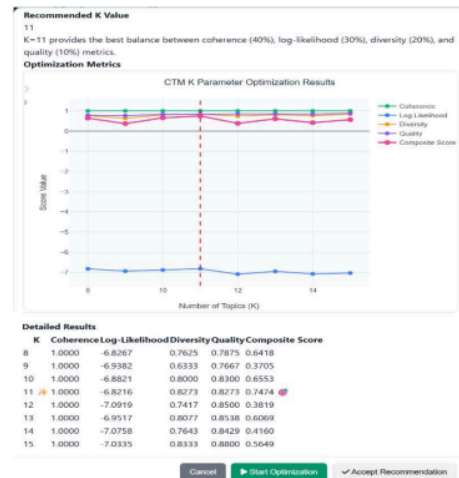
Gambar 4. 18 Output nilai optimasi K dan grafik nilai dari optimasi
