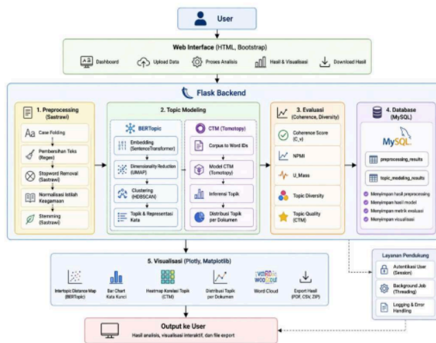
87 Gambar 4.13 Arsitektur Sistem
